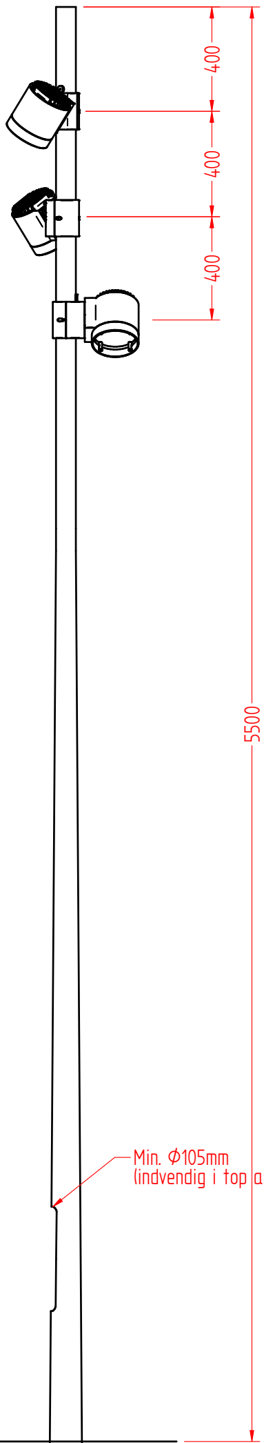
5,5 m mast: 3,5 m konisk + 2 m forlængerrør, \phi 76 mm - for 3 armatur
