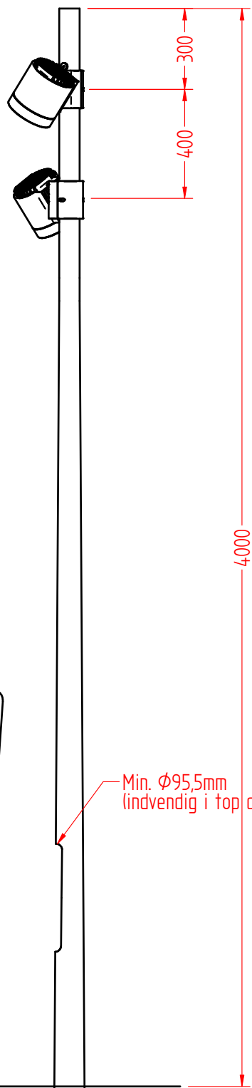
4 m mast: 3 m konisk + 1 m forlængerrør, \phi 76 mm - for 2 armatur
