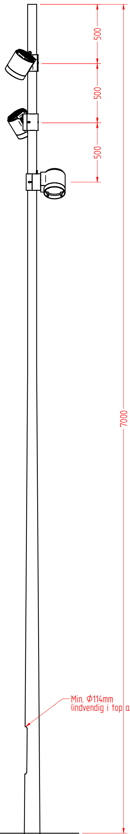
7 m mast: 4 m konisk + 3m forlængerrør, \phi 76 mm - for 3 armatur
